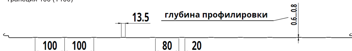
Рисунок 18. Виды профилировки наружной стороны сэндвич-панелей ПСТ Z
