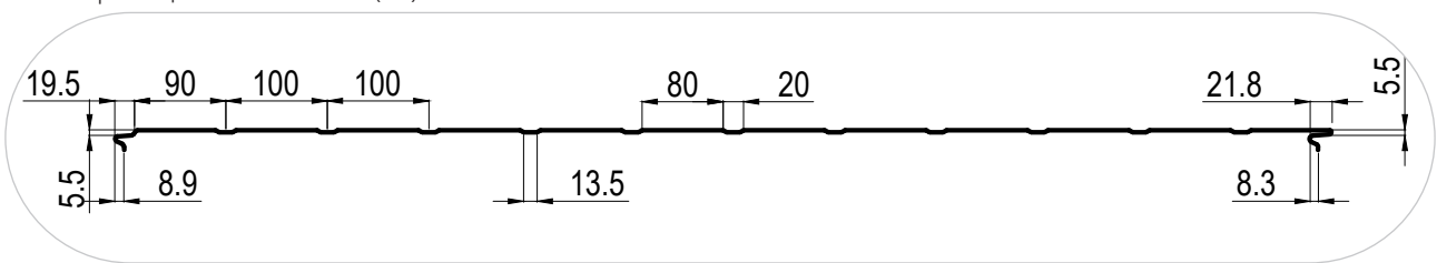
Рисунок 17. Виды профилировки внутренней стороны сэндвич-панелей ПСТ Z
