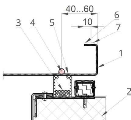
Рисунок 15: Схема расположения провода ПЭН в накладной раме
