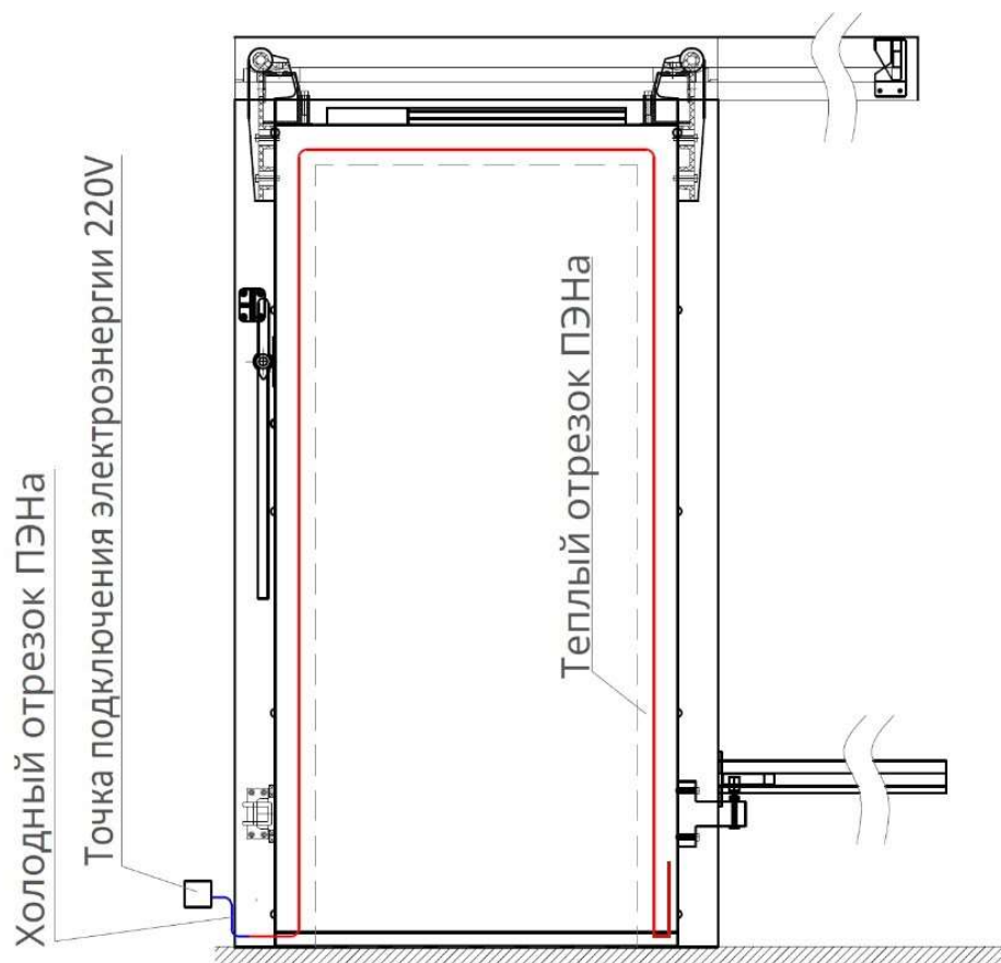
Рисунок 15: Схема расположения провода ПЭН в накладной раме
