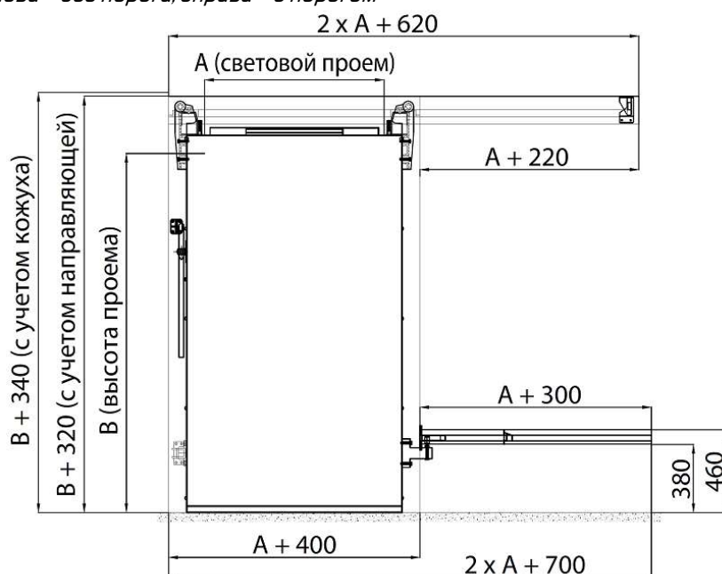
Рисунок 2. Металлическая накладная рама для дверей ОД П
