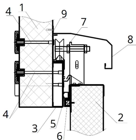
Рисунок 5. Крепление верхней направляющей и защитного кожуха к стене из сэндвич-панелей. Сечение в участке проема.
