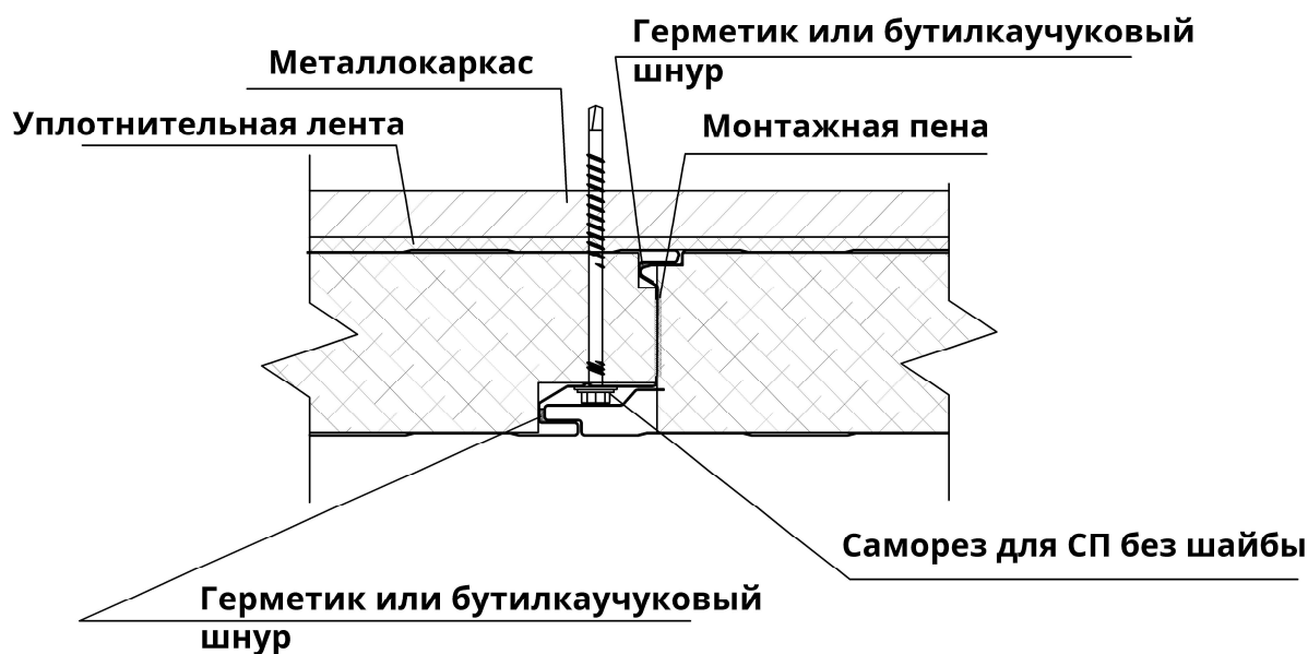
Рисунок 8. Замок стеновых панелей
