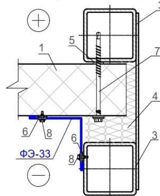
Горизонтальный разрез
