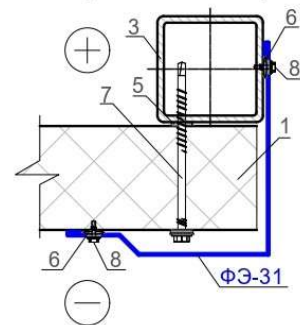
Горизонтальный разрез
