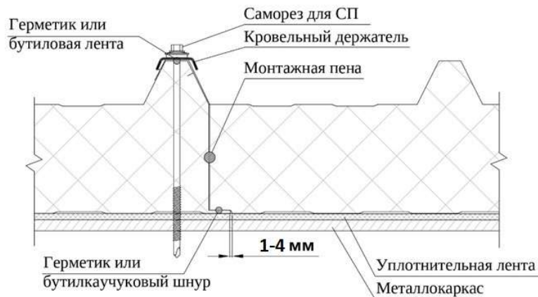
Рисунок 10. Замок кровельных панелей
