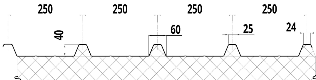
Рисунок 1-2. Геометрия кровельной сэндвич-панели с соединением Z-Lock.
