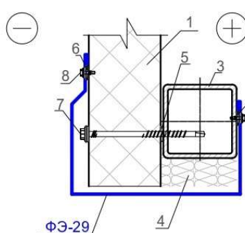
Вертикальный разрез
