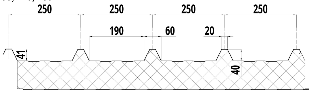
Рисунок 1-1. Геометрия кровельной сэндвич-панели со стандартным замковым соединением.
