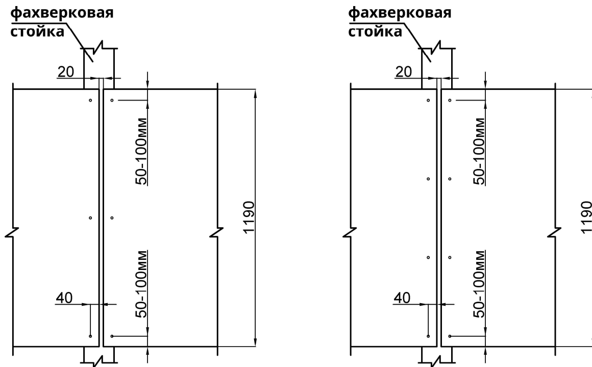
Рисунок 12. Стеновые панели ПСТ второго и последующих рядов. Варианты крепления к колонне или фахверку при горизонтальной раскладке.
