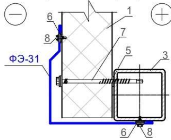
Вертикальный разрез
