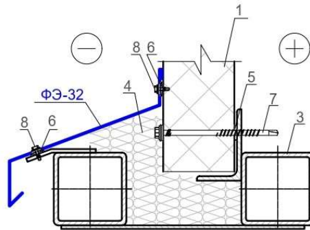
Вертикальный разрез
