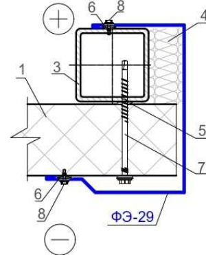
Горизонтальный разрез
