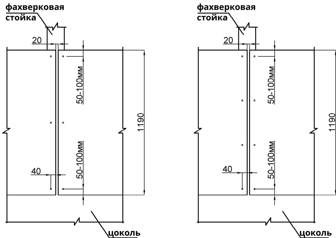
Рисунок 11. Стеновые панели ПСТ первого ряда. Варианты крепления к колонне или фахверку при горизонтальной раскладке.
