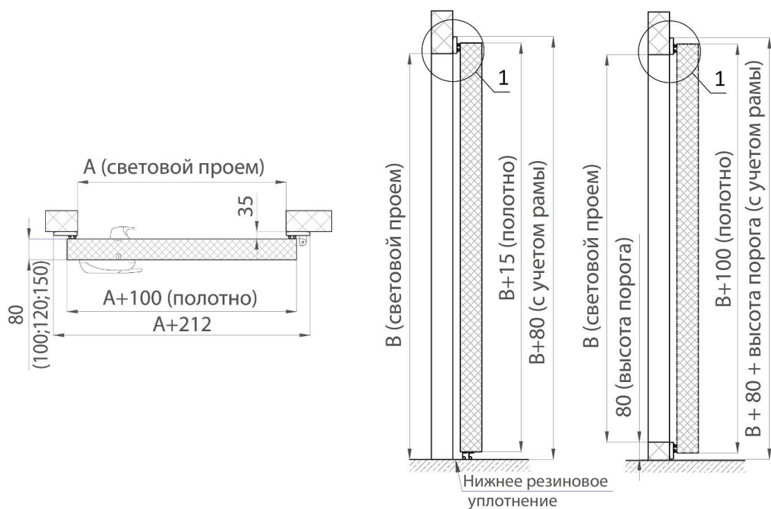
Рисунок 4. Разрез А-А.
