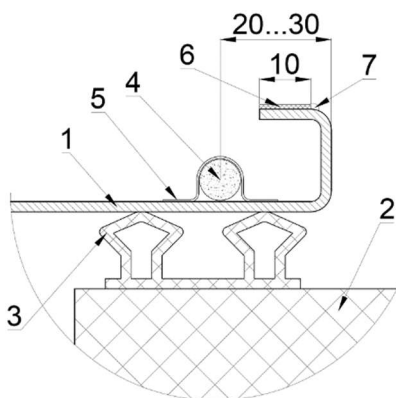
Рисунок 10. Узел 3. Крепление ПЭНа
