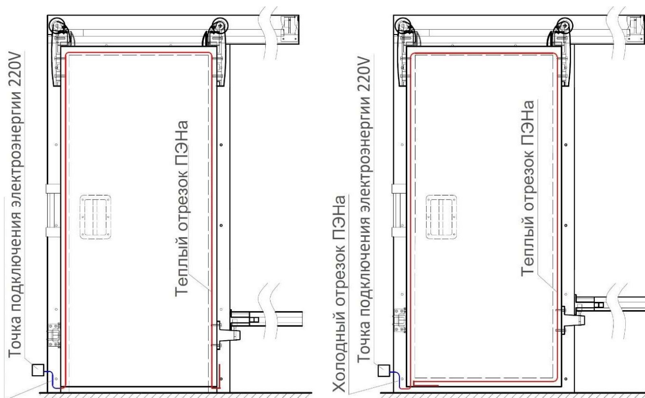
Рисунок 15: Схема расположения провода ПЭН в накладной раме Слева – исполнение рамы без порога; справа – с порогом
