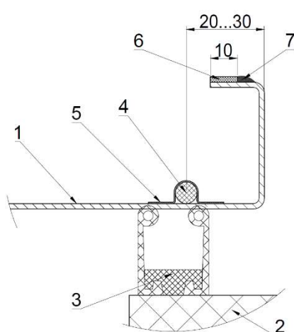
Рисунок 16. Узел крепления ПЭНа на раме
